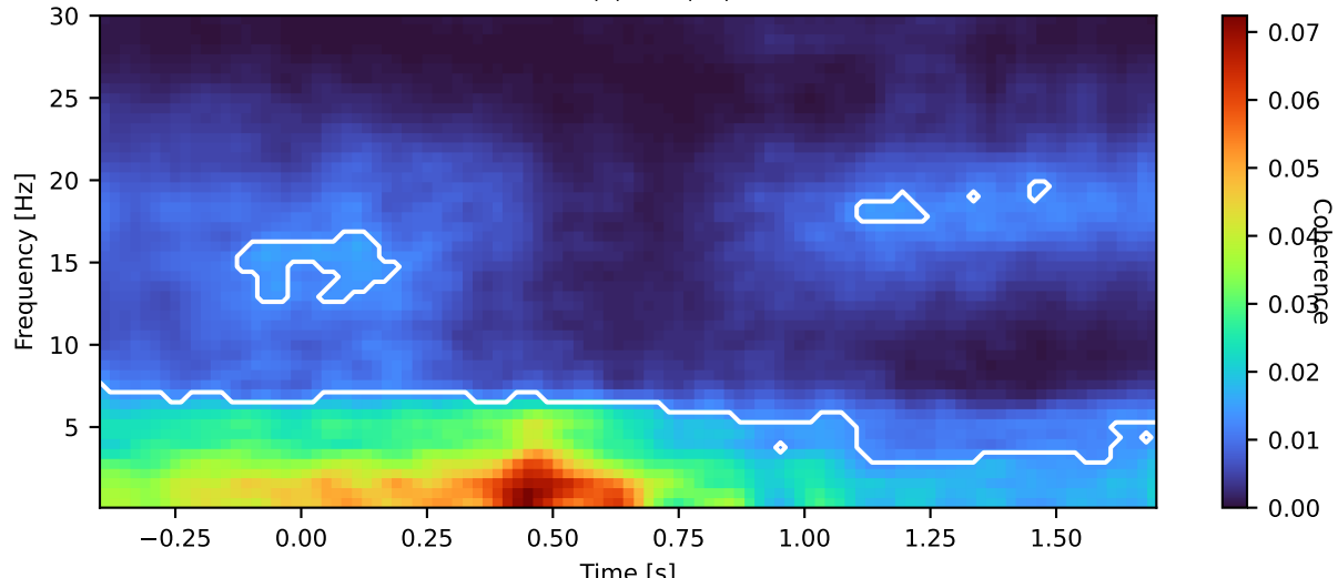
dPFC (6) - PE (12)
